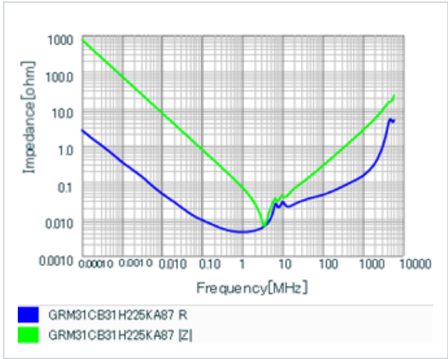
■ 周波数特性 (ESR、Impedance)
